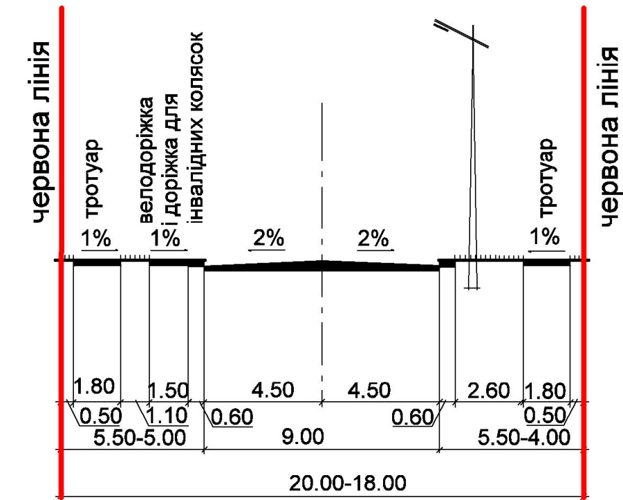
Розріз II-II
