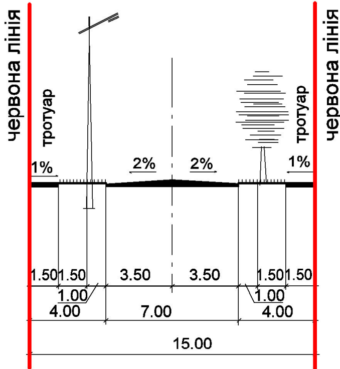
Розріз III-III
