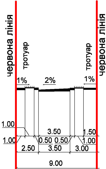
Розріз V-V
