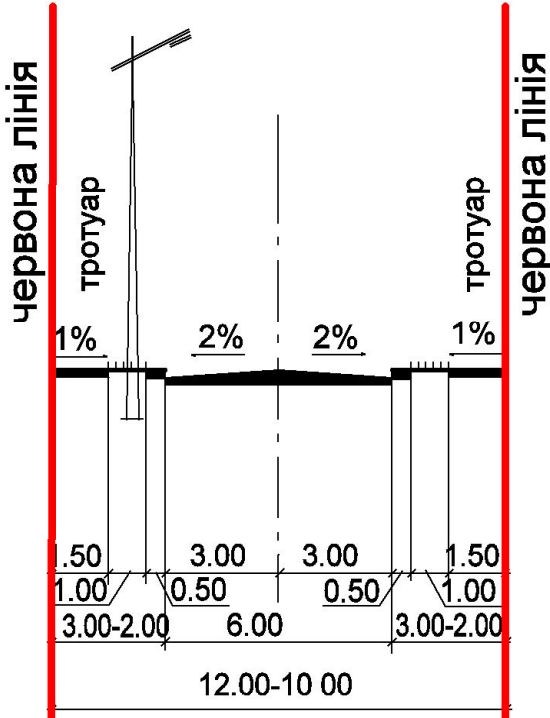
Розріз IV-IV
